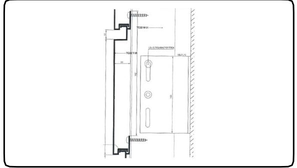
004 FUGALI PROFİL CEPHE KAPLAMA DETAYI
