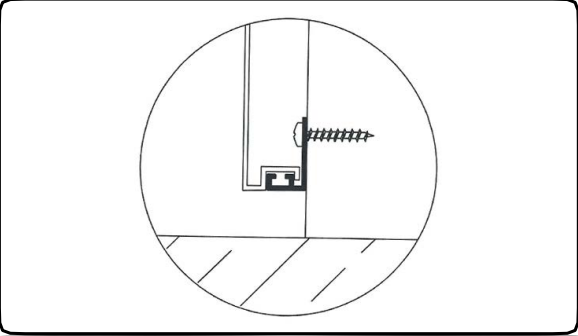
003 BAŞLANGIÇ PROFİL DETAYI
