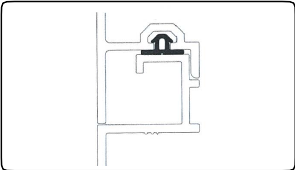
005 FUGASIZ PROFİL CONTA DETAYI
